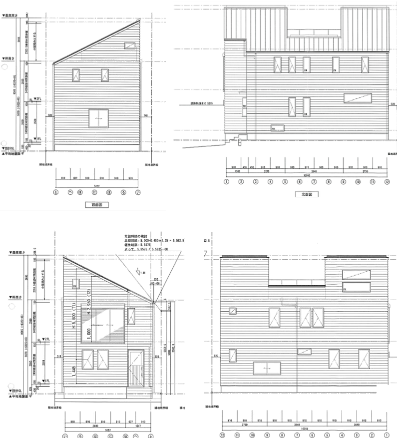
立面図
