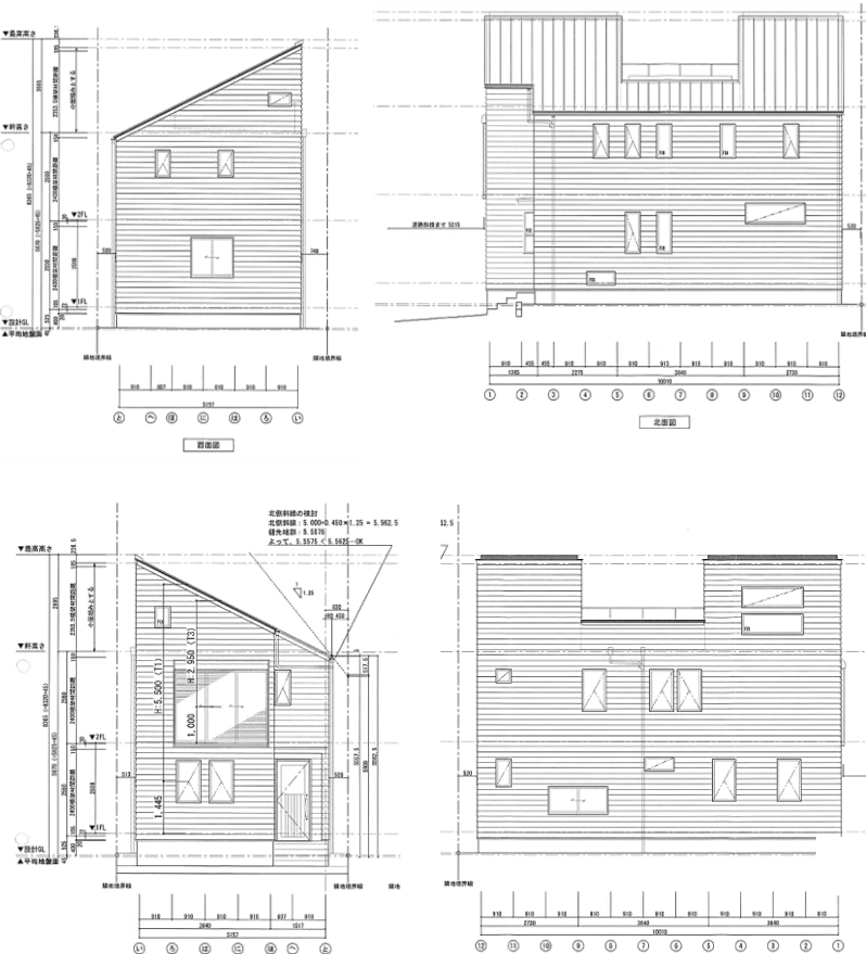
立面図
