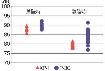
図1 滑走路北約1線におけるXP-1とP-3Cの最高音
