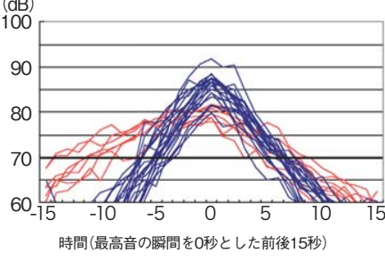
図2 滑走路北約1線におけるXP-1とP-3Cの騒音の波形(離陸時)
