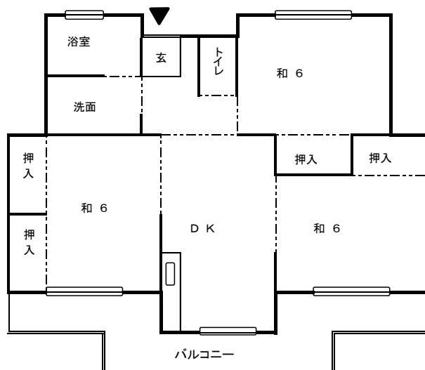
間取り図
