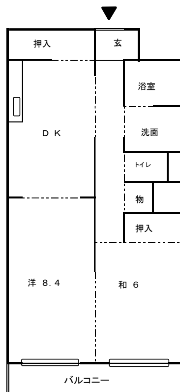
間取り図
