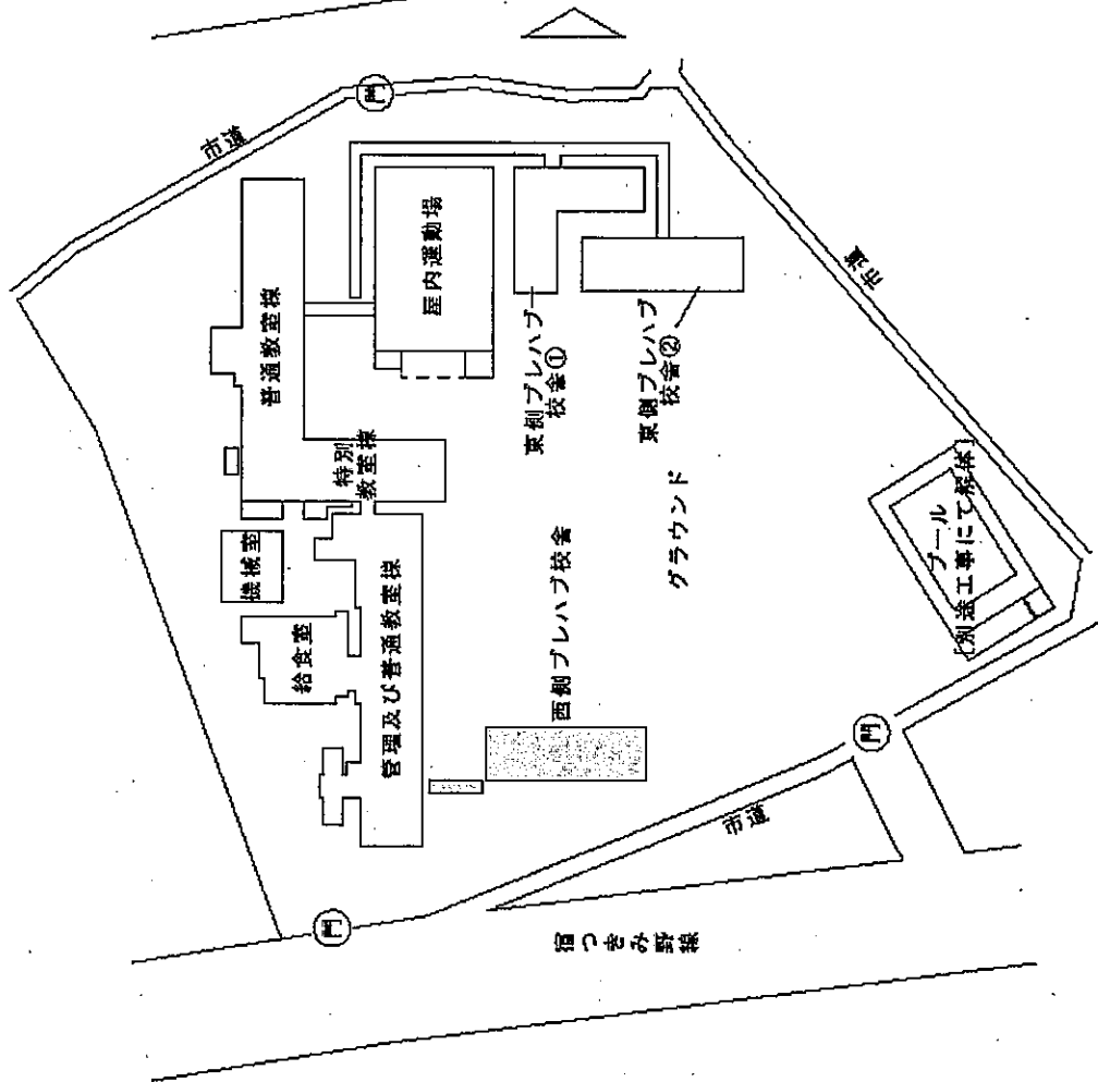
現況配置図
