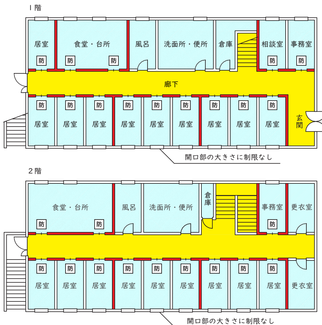
別図2 省令第12条の2第1項第1号
