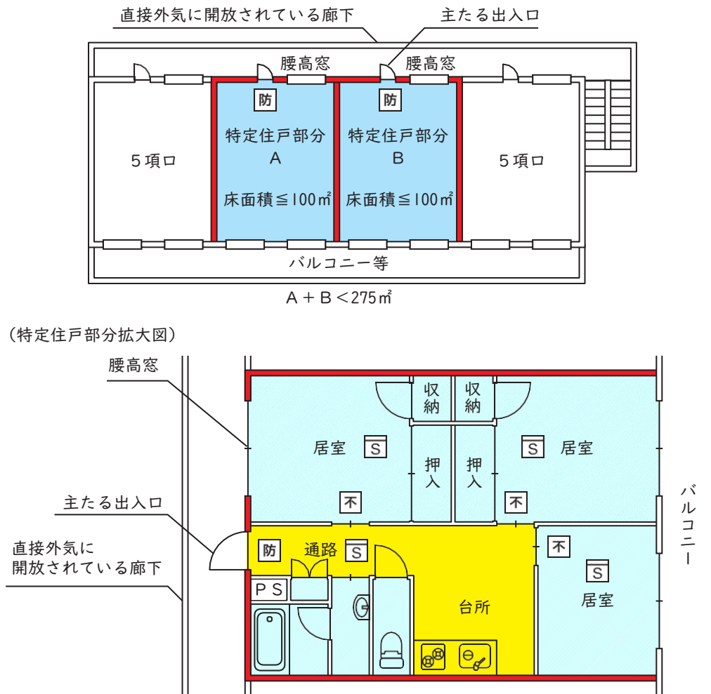
別図6 省令第12条の2第3項
