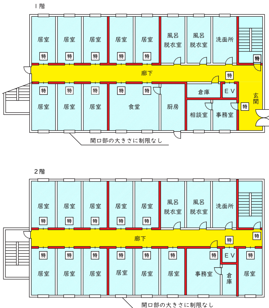
別図3 省令第12条の2第1項第2号
